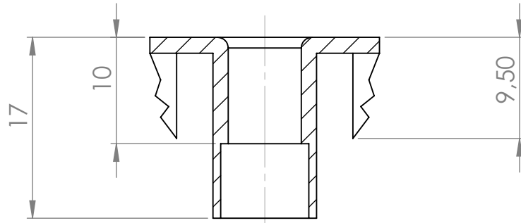
KESIT D-D
